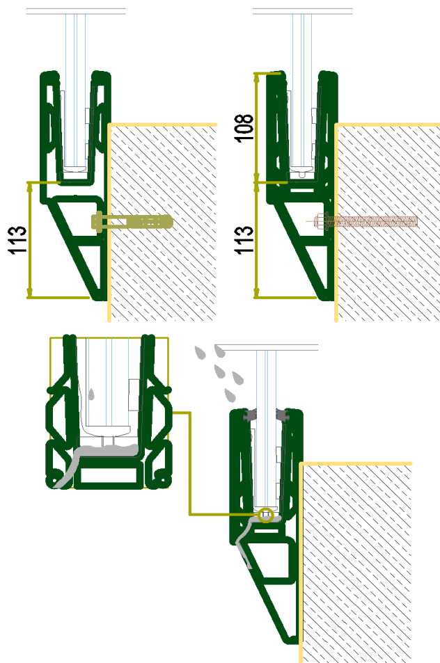
Détail Profil KF1200 (Fixation non testée)
